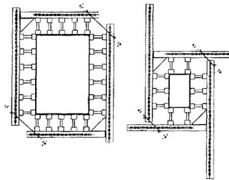
Рисунок 2.5 - Бесступенчато изменяемая опалубка для колонн «ВАРИО»
