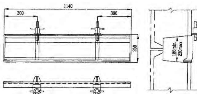
Рисунок 2.22 - Опалубка для бетонирования вертикальных стыков
