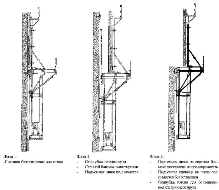
Рисунок 2.4 - Последовательность тактов подъема опалубки «Пари ACS-50»
