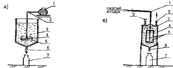
Рисунок 2.24 - Смесители для приготовления смазок
