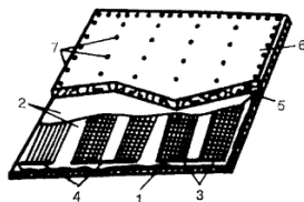
Рисунок 5.2 - Сетчатый нагреватель
