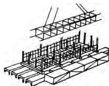
Рисунок 3.4 Кондуктор-шаблон для сборки каркасов
