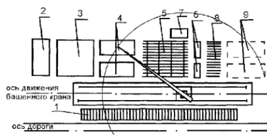
Рис. 3.3 - Организация сборочно-комплектующей площадки для сборки арматурно-опалубочных блоков:
