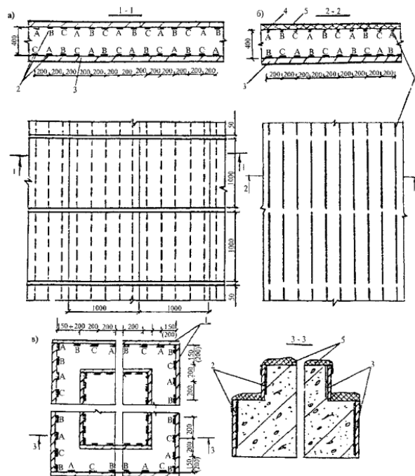
Рисунок К.3 - Расстановка и расфазировка электродов
