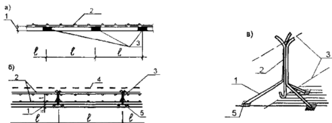
Рисунок 3.1 - Фиксаторы защитного слоя бетона для горизонтальной арматуры:
