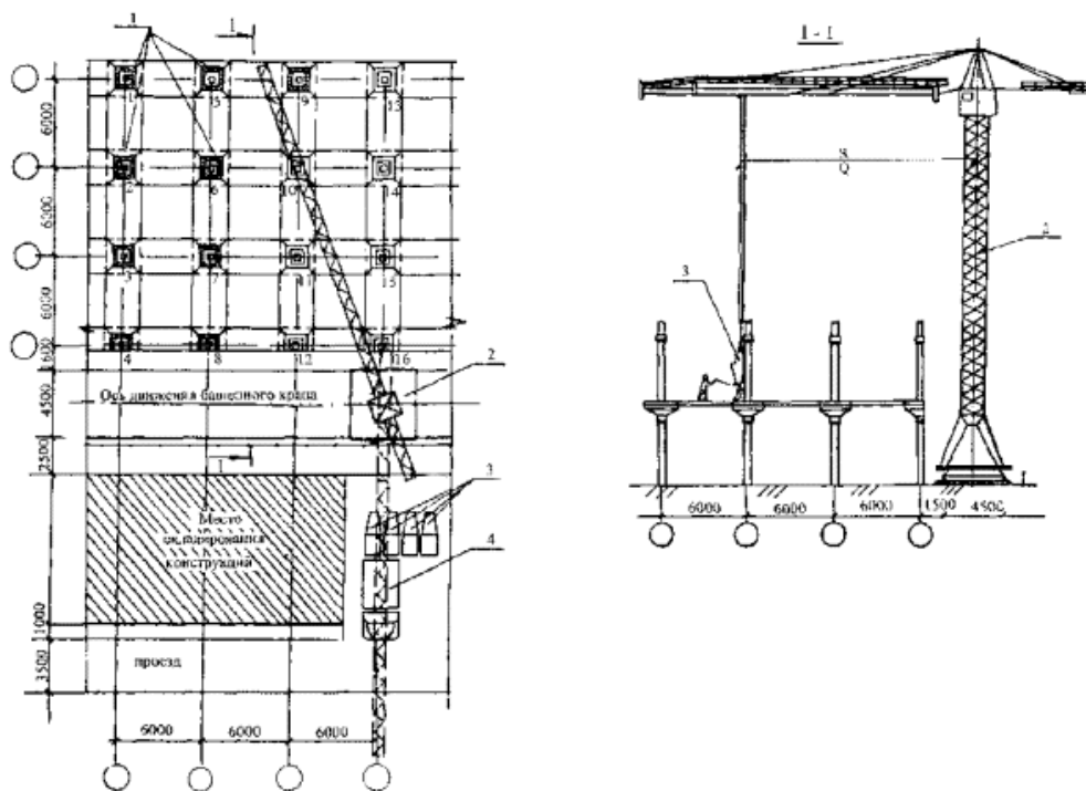
Рисунок 7.15 - Технологическая схема замоноличивания полости капители
