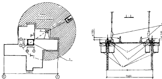
Рисунок 7.10 - Схема бетонирования ядра жесткости на строительстве общежития АОН
