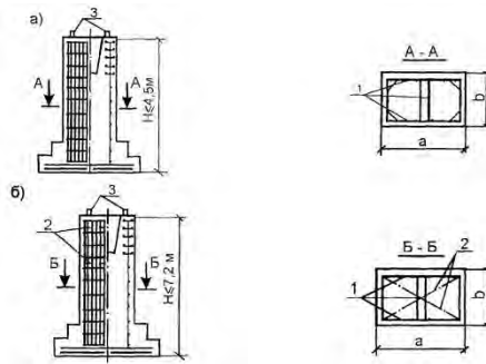
Рисунок 3.6 - Армирование фундаментов колонн пространственными самонесущими арматурными каркасами, собираемыми из плоских сеток
