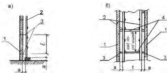
Рисунок 3.2 - Фиксаторы защитного слоя бетона для вертикальной арматуры:
