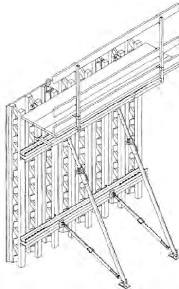
Рисунок 2.1 - Система «ПЕРИ Варио цугфест» - балочная опалубка для бетонирования стен
