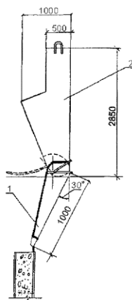
Рисунок 4.2 - Направляющий лоток бункера для бетонирования тонкостенных монолитных конструкций
