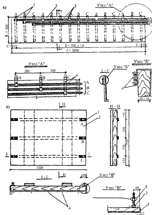
Рисунок К.2 - Расстановка и расфазировка полосовых электродов
