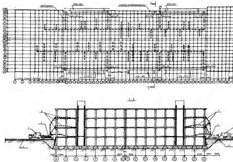
Рисунок 7.9 - Схема устройства бетонных полов универсального хранилища Краснопресненской плодовоощной базы
