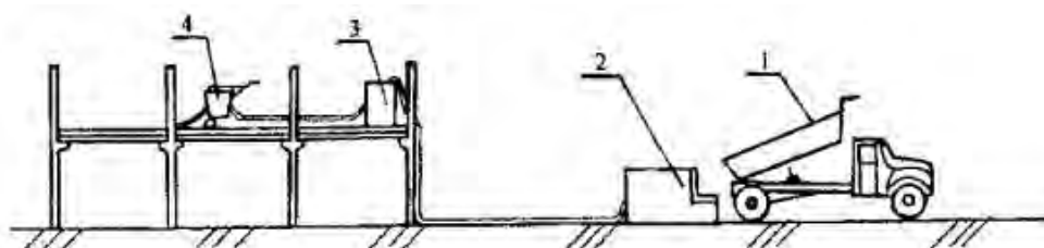
Рисунок 7.17 - Схема замоноличивания стыков с подачей раствора растворонасосной установкой
