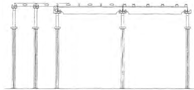
Рисунок 2.6 - Опалубка системы «Пери Скайдек»
