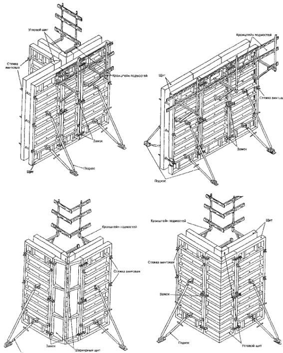
Рисунок 2.20 - Алюминиевая опалубка стен
