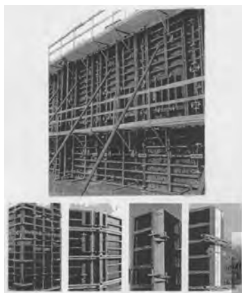
Рисунок 2.8 - Опалубка системы «Маммут»
