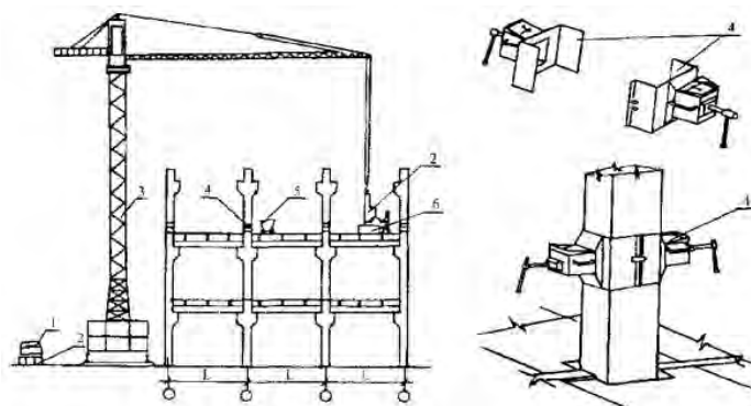
Рисунок 7.16 - Схема замоноличивания стыков колонн с помощью пресс-опалубки
