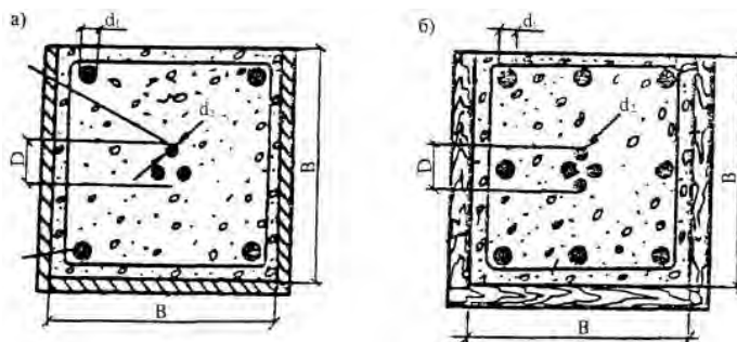
Рисунок К.1 - Схема размещения струнных электродов при прогреве конструкций квадратного сечения:
