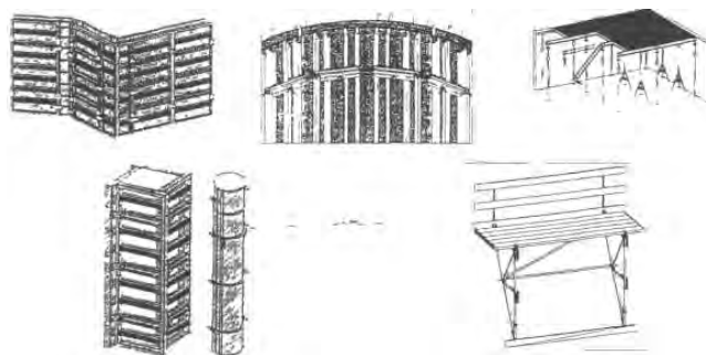
Рисунок 2.23 - Варианты использования комплектной опалубки «НОЕ»
