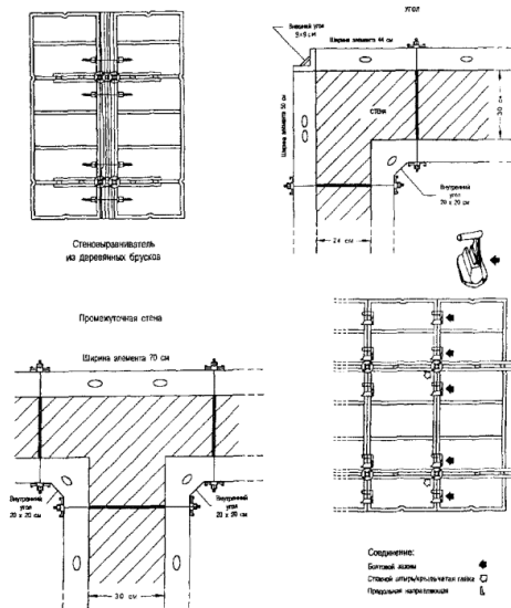
Рисунок 2.12 - Схемы установки опалубки «Далли»
