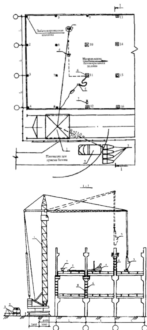
Рисунок 7.4 - Схема бетонирования колонн с помощью башенного крана КБ-160.2
