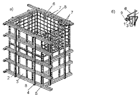
Рисунок 3.7 - Арматурно-опалубочный блок
