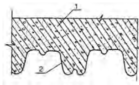
Рисунок 2.14 - Несъемная опалубка из профилированного настила
