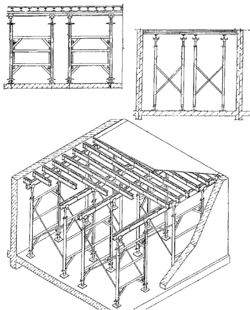
Рисунок 2.21 - Алюминиевая опалубка перекрытий
