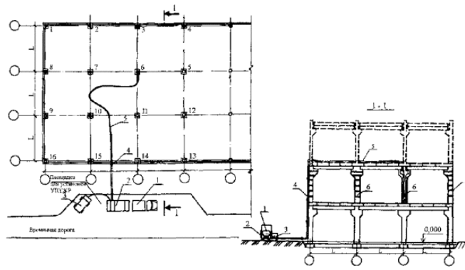
Рисунок 7.5 - Схема обетонирования колонн с применением УПТЗР
