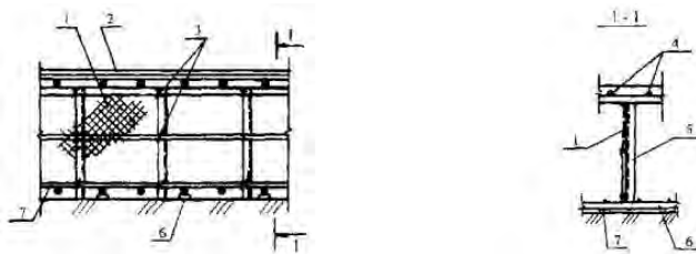
Рисунок 7.1 - Конструкция рабочего шва
