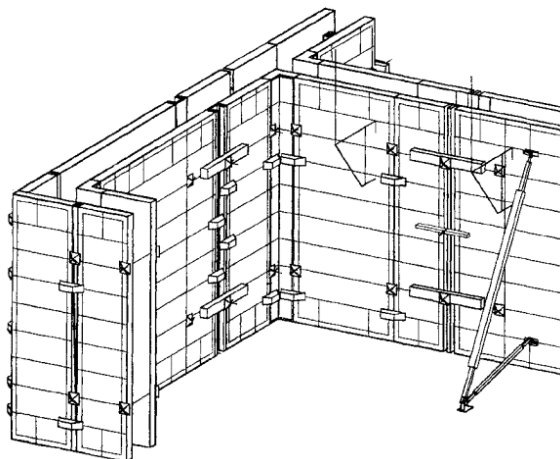
Рисунок 2.3 - Система «Пери Трио»
