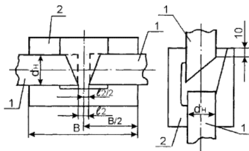
Рисунок 3.8 - Установка инвентарной формы на свариваемые арматурные стержни:
