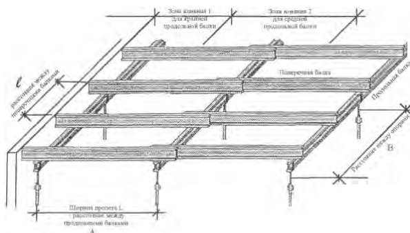
Рисунок 2.18 - Схема укладки металлодеревянных балок ОПРУС 250 (300, 360)
