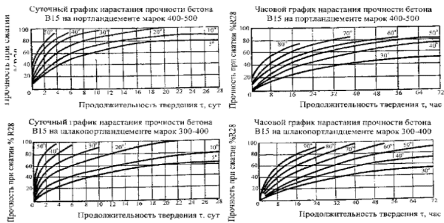
Рисунок Г.1 - Графики нарастания прочности бетона при различных температурах бетонной смеси
