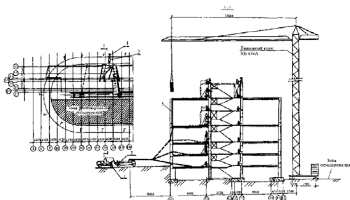
Рисунок 7.11 - Схема бетонирования ядра жесткости автобетононасосом «Штеттер» (учебный корпус комплекса зданий МВТУ им. Баумана)
