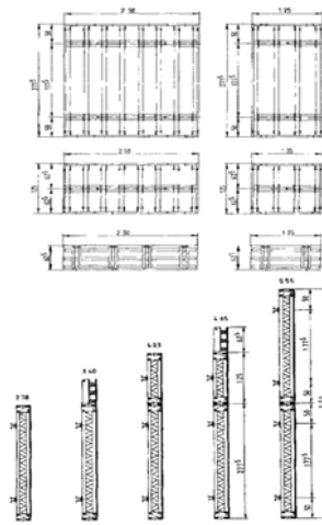
Рисунок 2.2 - Опалубка системы «ВАРИОФИКС», наращиваемая растром 60 см
