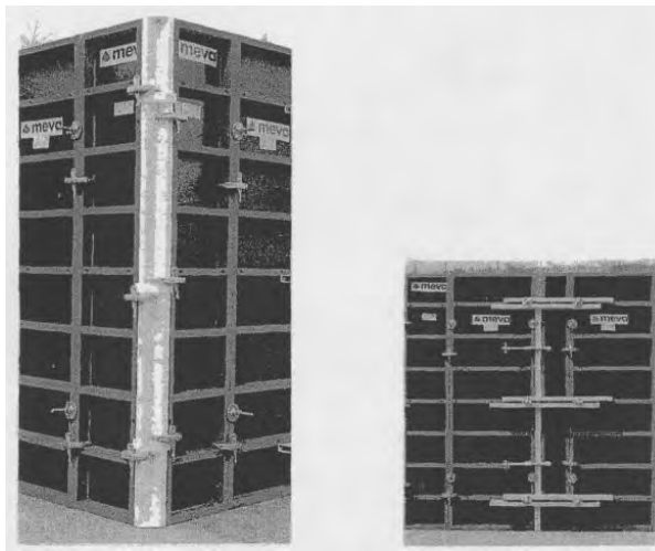
Рисунок 2.7 - Опалубка системы «Стар Тек»
