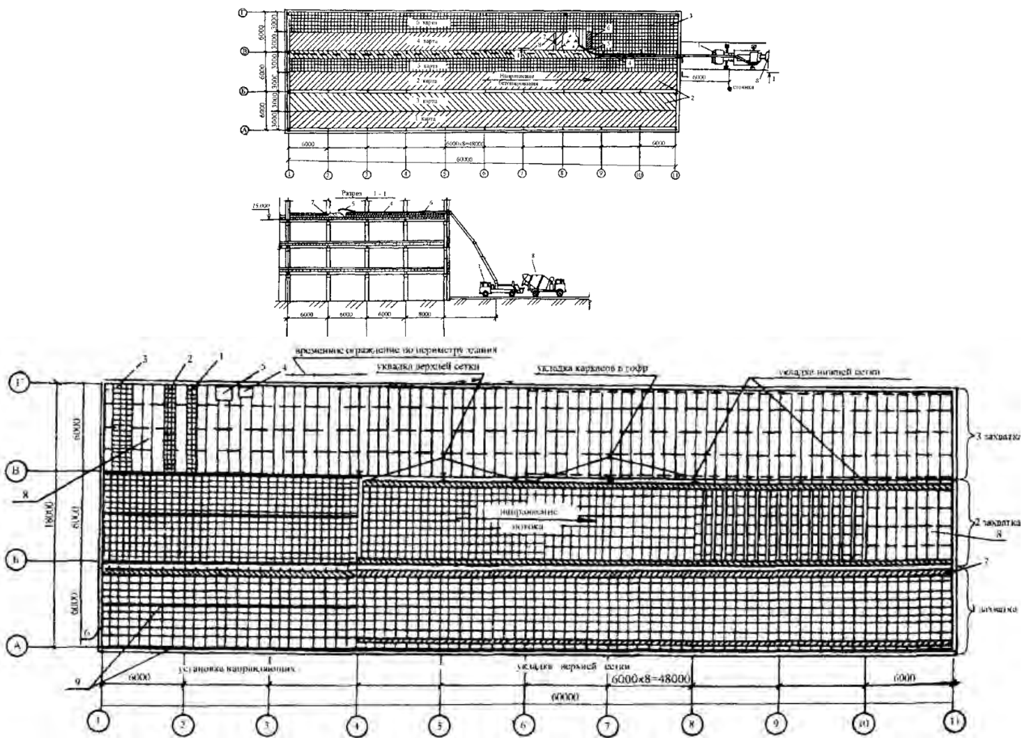
Рисунок 7.6 - Технологическая схема армирования монолитных перекрытий с применением профнастила
