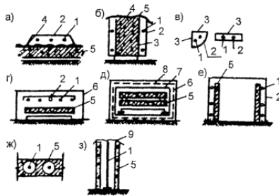
Рисунок 5.1 - Некоторые модификации установок инфракрасного нагрева закрытого типа
