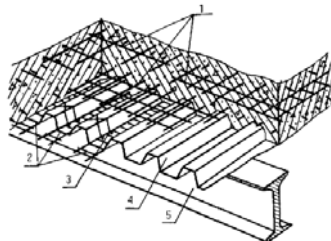
Рисунок 2.13 - Конструкция монолитного перекрытия с применением стального профилированного настила
