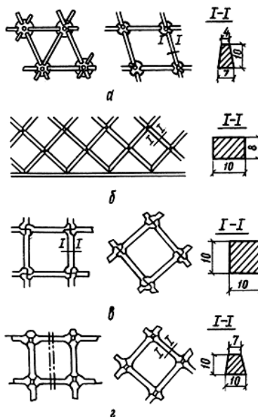
Рис. 1. Варианты компоновки элементов решетчатых конструкций
