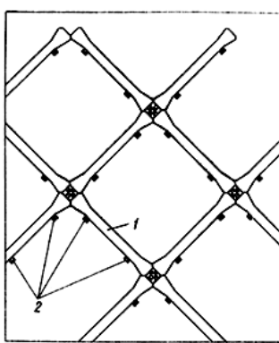
Рис. 3. Временное крепление узлов решетки при монтаже
