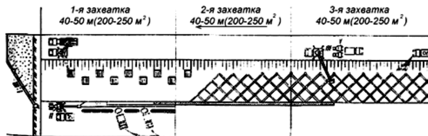
Рис. 2. Схема организации и производства работ
