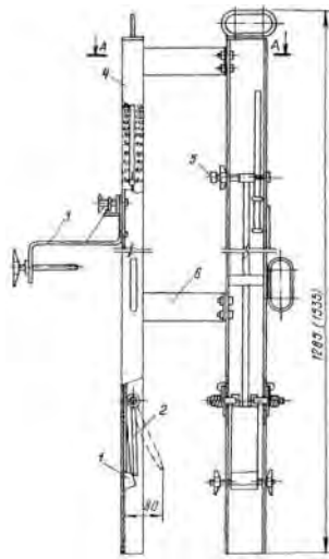
Инвентарный фиксатор
