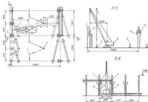
Схема монтажа подкрановых балок
