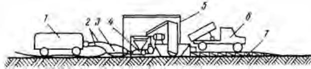
Схема заделки стыков при приготовлении песчаной бетонной смеси на стройплощадке
