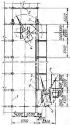
Ячейка здания пролетом 12 м, шаг колонн и стропильных конструкций 6 м
