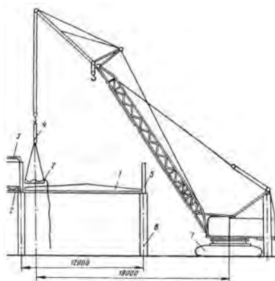
Укладка плиты
