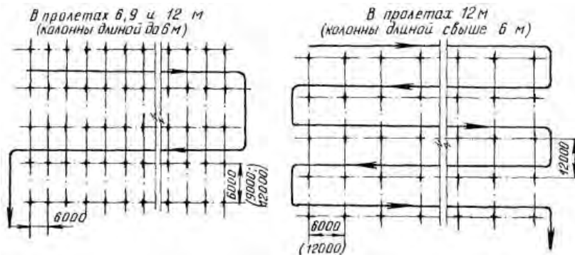
Схемы движения крана при установке колонн
