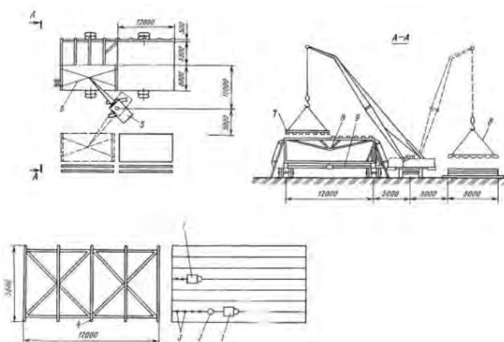
Схема монтажа покрытия из профилированного настила
