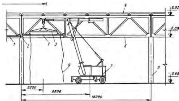
Укладка плиты
