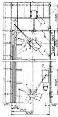
Шаг колонн и ферм 12 м
