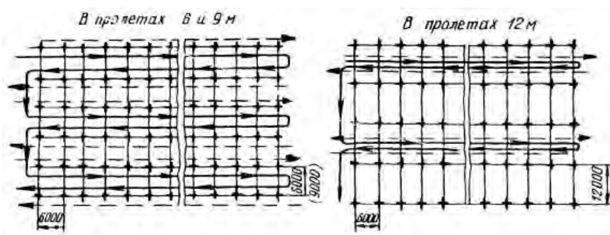
Схемы движения крана и автомобиля при раскладке колонн
