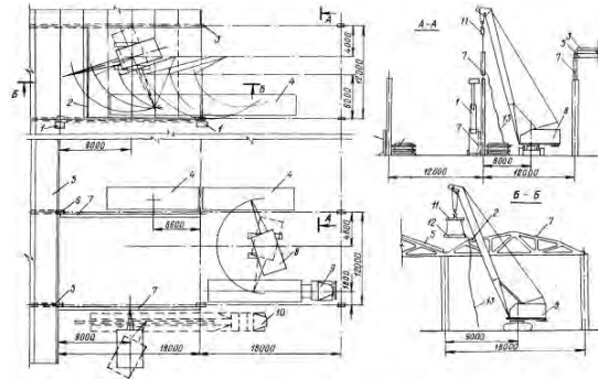
Схемы выгрузки, раскладки элементов и монтажа поперечным методом покрытия пролетом 18 м
