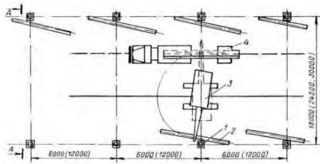
Схема движения крана и автомобиля
