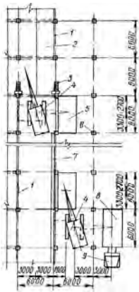
Ячейка здания пролетом 9 м, шаг колонн и стропильных конструкций 6 м
