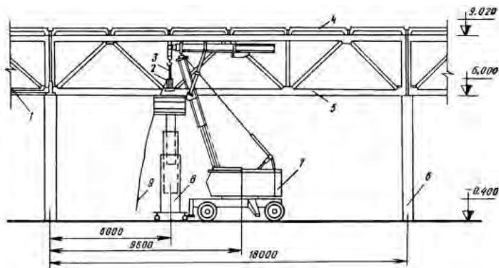
Укладка плиты
