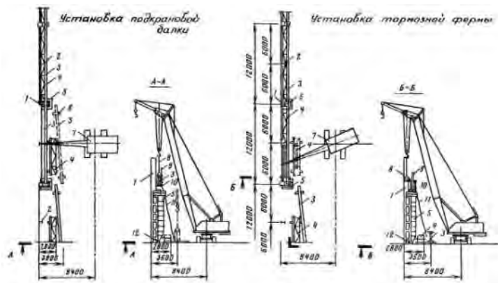
Схема монтажа подкрановых балок пролетом 12 м отдельными элементами по колоннам крайнего ряда со стойками фахверка
