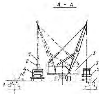
Схема установки колонн
