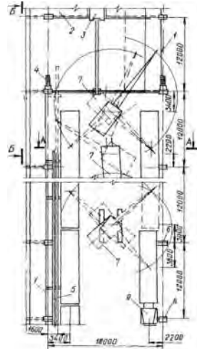
Шаг колонн и ферм 12 м
