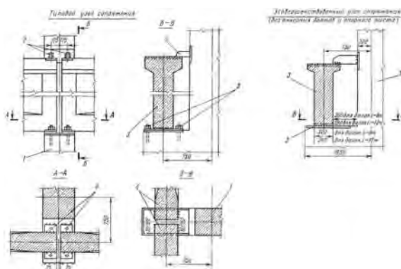
Детали опирания подкрановых балок на среднюю колонну
