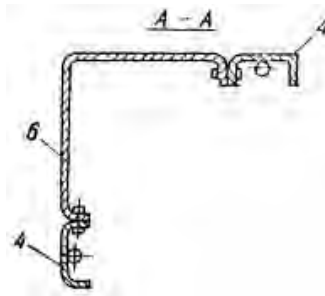
Инвентарный фиксатор
