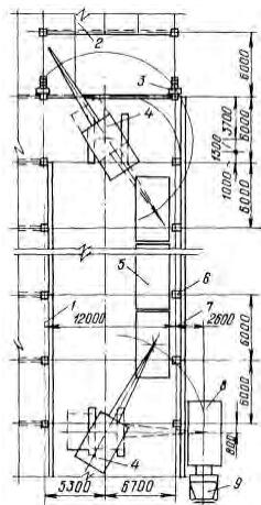
Ячейка здания пролетом 12 м, шаг колонн и стропильных конструкций 6 м
