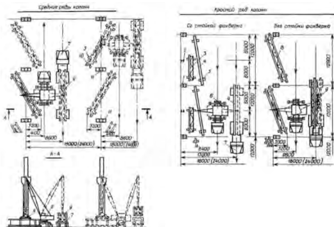
Схема выгрузки и раскладки укрупненных блоков подкрановых балок пролетом 12 м
