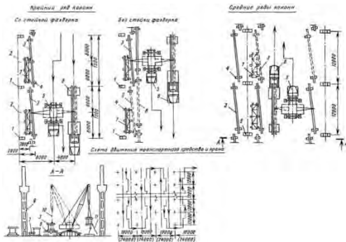
Схема выгрузки и раскладки подкрановых балок пролетом 12 м при установке их отдельными элементами
