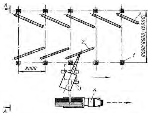
Схемы движения крана и автомобиля при раскладке колонн
