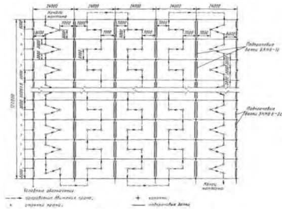
Схема монтажа подкрановых балок
