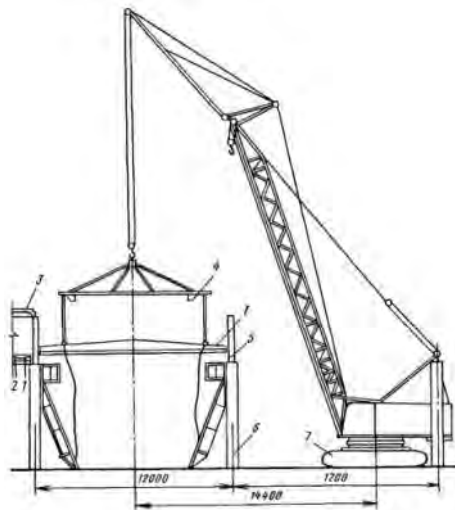
Укладка плиты
