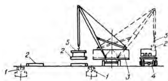
Выгрузка и предварительная раскладка колонн в зданиях пролетами 18, 24 и 30 м
