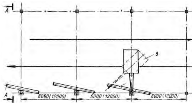
Схемы движения крана при установке колонн
