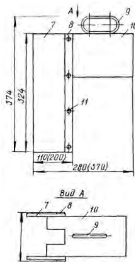
Ограждение клинового вкладыша
