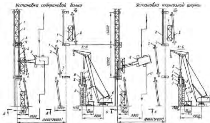
Схема установки подкрановых балок пролетом 12 м отдельными элементами по колоннам среднего ряда
