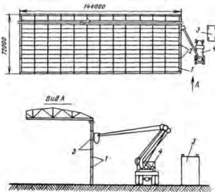
Схема расположения оборудования при герметизации стыков панелей наружных стен
