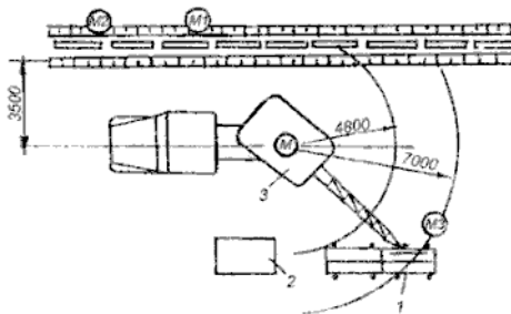
Рис.2. Организация рабочего места
