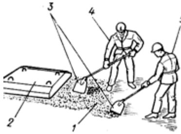
Рис.11. Схема подготовки песчаного основания:
