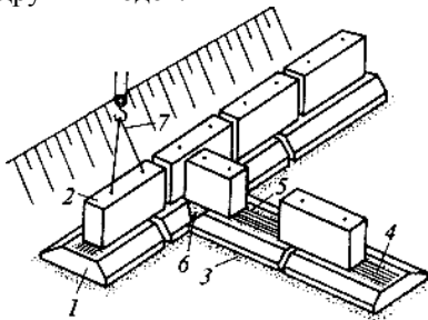
Рис.1. Монтаж сборных ленточных фундаментов:
