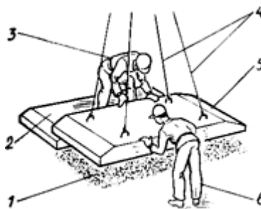
Рис.12. Схема установки сборного фундаментного блока:
