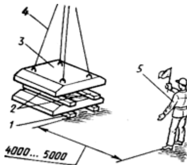
Рис.10. Схема подъема сборного блока фундаментов:
