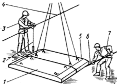
Рис.13. Схема выверки устанавливаемого блока:
