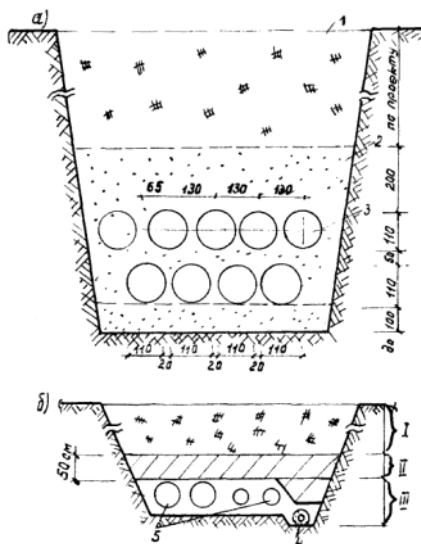
Рис. 4.3. Схема обратной засыпки траншей:
