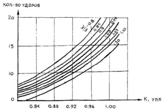
График 2. Определение коэффициента уплотнения супесей
