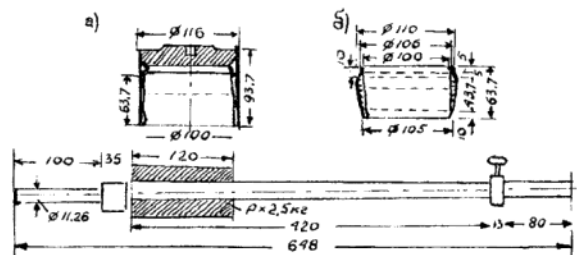
Рис. 1. Грунтоотборник:
