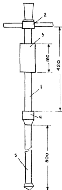
Рис. 1. Прибор ДПУ для контроля плотности грунта
