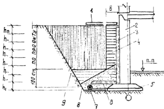
Рис. 3.1. Схема обратной засыпки пазухи котлована:
