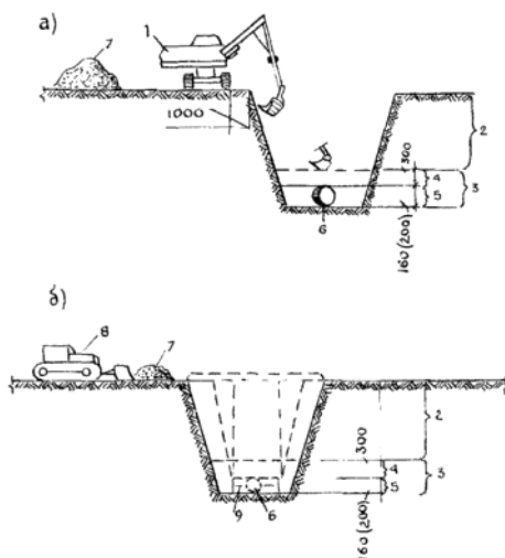
Рис. 4.2. Схема организации работ по засыпке траншей:
