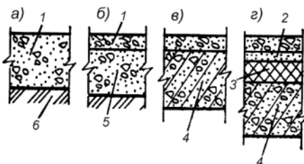
Рис.1. Бетонные полы
