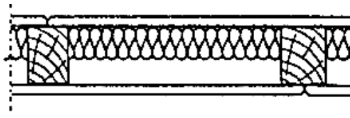
Рис.28. Стена с деревянным каркасом (С121)
