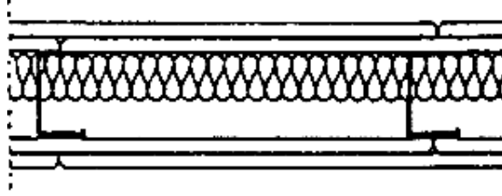
Рис.25. Стена с металлическим каркасом (С112)
