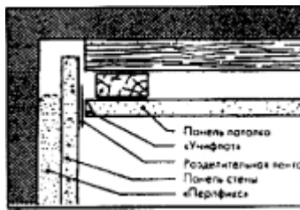
Рис.21. Гипсовые панели стены и подвесного потолка
