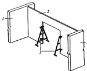
Рис.11. Схема временного крепления железобетонной перегородки:
