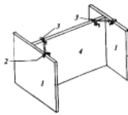
Рис.9. Схема крепления панели внутренней стены с помощью двух монтажных связей: 1 - закрепленная панель внутренней стены; 2- инвентарная петля; 3 -монтажная связь; 4- монтируемая панель внутренней стены
