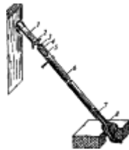
Рис.4. Подкос с трехсторонним захватом для временного крепления наружных стеновых панелей:
