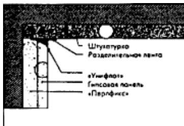
Рис.20. Гипсовая панель стены и штукатурка потолка
