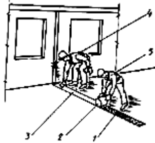
Рис.16. Схема расстилания гидроизолирующего слоя
