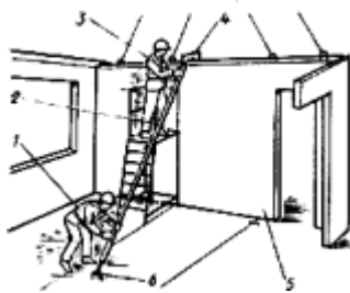
Рис.18. Схема закрепления сборного элемента
