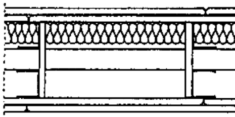
Рис.27. Стена с металлическим каркасом (С116)
