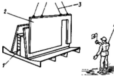
Рис.14. Схема подъема элемента
