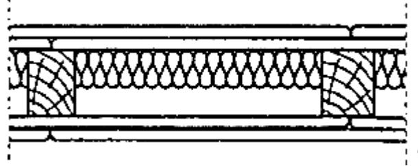
Рис.29. Стена с деревянным каркасом (С122)
