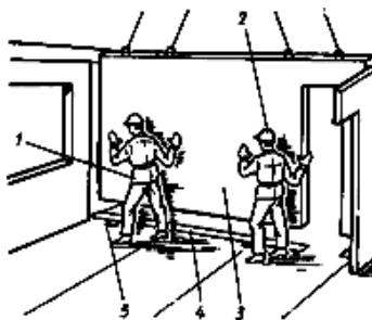
Рис.17. Схема установки сборного элемента
