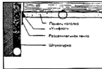
Рис.23. Гипсовая панель подвесного потолка и штукатурка стены
