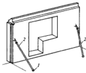
Рис.3. Схема временного крепления панели наружной стены: 1 - технологическое отверстие; 2 -подкос для монтажа панелей наружных стен
