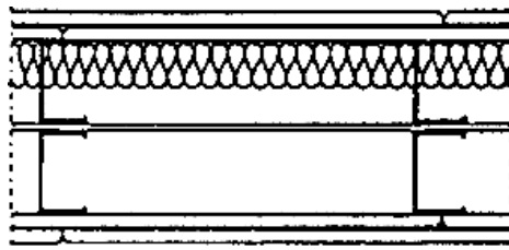
Рис.26. Стена с металлическим каркасом (С115)
