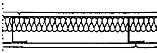
Рис.24. Стена с металлическим каркасом (С111)
