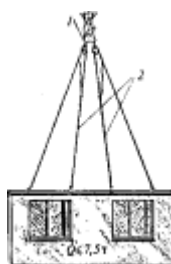
Рис.2. Строповка и подъем стеновой панели за четыре подъемные петли:
