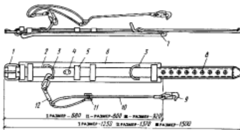
Рис.12. Предохранительный пояс:
