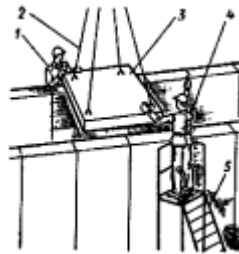
Рис.4. Схема укладки лестничной площадки
