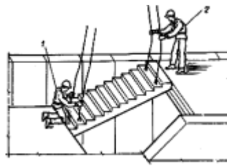
Рис.10. Схема расстроповки лестничного марша
