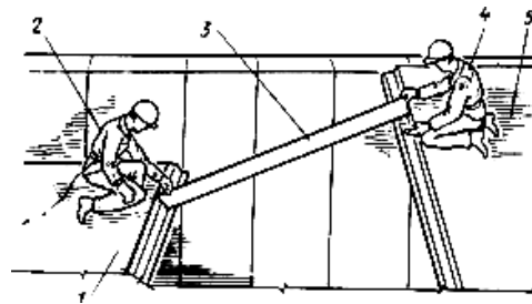
Рис.5. Схема выверки лестничной площадки
