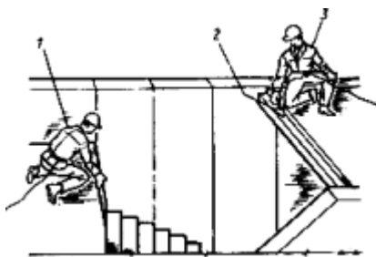
Рис.7. Схема подготовки места установки лестничного марша
